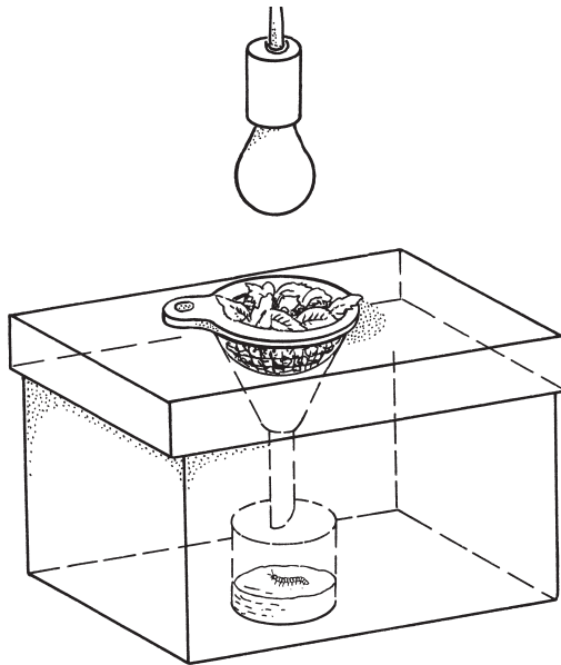
Berlesetrichter
